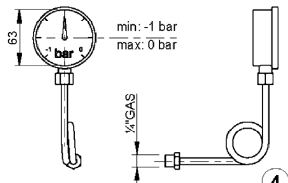
VUOTOMETRO VACUUM GAUGE
