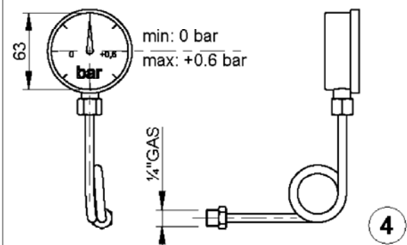
MANOMETRO PRESSURE GAUGE
