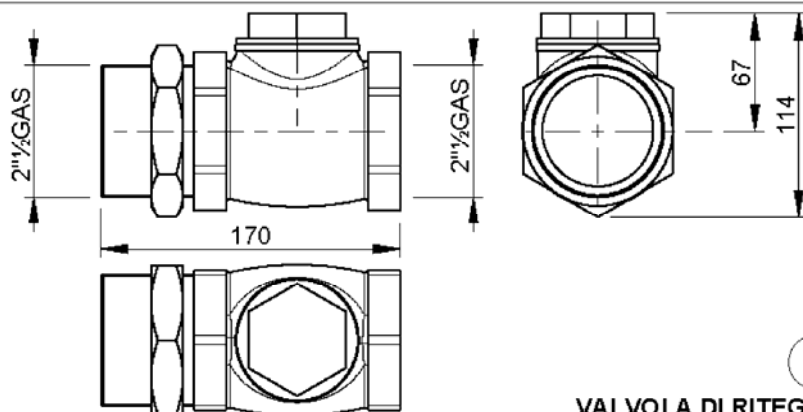
VALVOLA DI RITEGNO NON RETURN VALVE tipo-type: VR8
