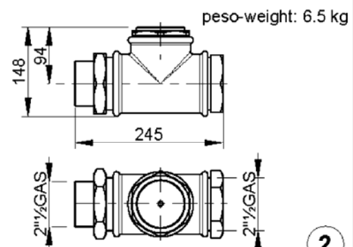
VALVOLA DI SOVRAPRESSIONE OVERPRESSURE RELIEF VALVE tipo-type: SV8/10T
