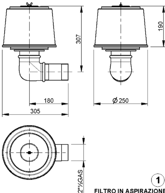
FILTRO IN ASPIRAZIONE INLET FILTER tipo-type: F10NGR8
